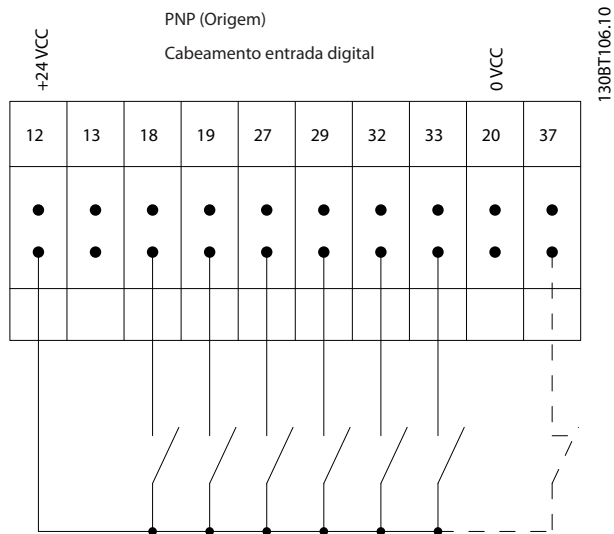
Ilustração 1.3 PNP (Origem)
