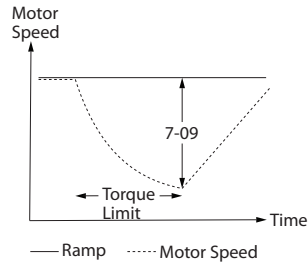
Ilustração 3.49 Erro de Velocidade entre Rampa e Velocidade Real
