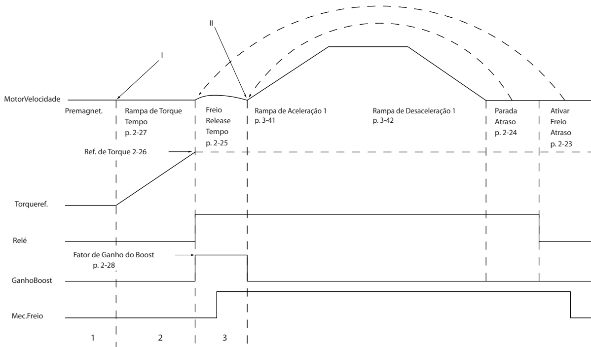
Ilustração 3.20 Sequência de liberação do freio para controle do freio mecânico do içamento. Esse controle de frenagem está disponível no princípio de controle de fluxo com feedback ou no modo sem sensor, disponível para motores assíncronos e motores PM não saliente.
