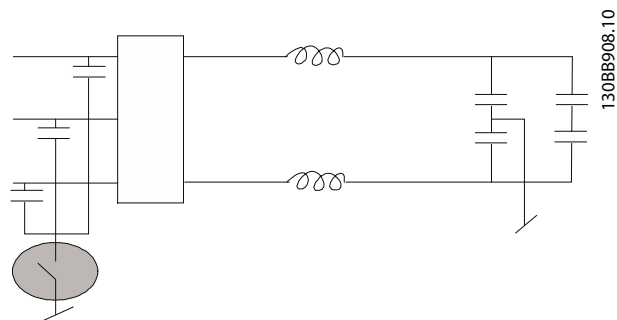
Ilustração 3.62 Filtro de RFI
