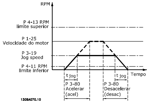
Ilustração 3.27 Tempo de Rampa do Jog
